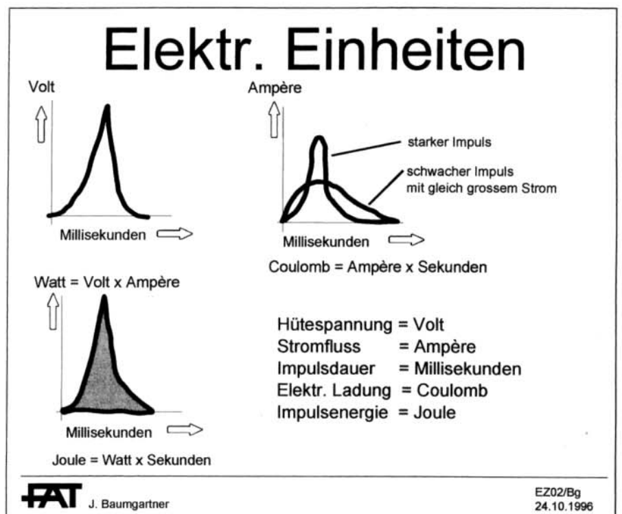
Abb. 4. Alle 1 bis 1,5 Sekunden gibt das Elektrozaungerät einen Impuls an den Zaun ab. Dieser besteht aus Strom und Spannung und dauert nur Millisekunden. Aus diesen Einheiten lassen sich die übrigen Beurteilungsgrössen berechnen.
