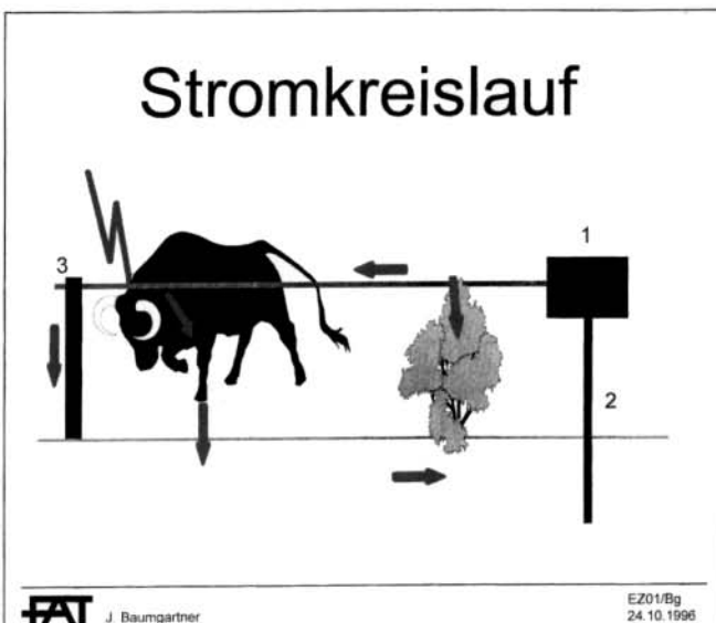
Abb. 2. Funktionsschema des Elektrozauns: Nur ein geschlossener Stromkreislauf garantiert eine hohe Hütessicherheit.
