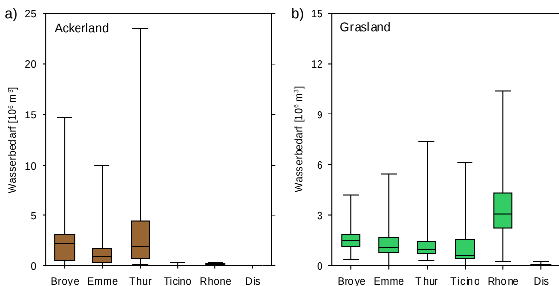
Abbildung 6: Gebietsbezogener saisonaler Bewässerungsbedarf (Spannweite, Median, 1.+ 3. Quartil) für Ackerflächen und Grasland (1980 - 2006), jeweils ermittelt nach ET/ETP-Schwellwertmethode (beachte unterschiedliche Skalierung der y-Achse).
