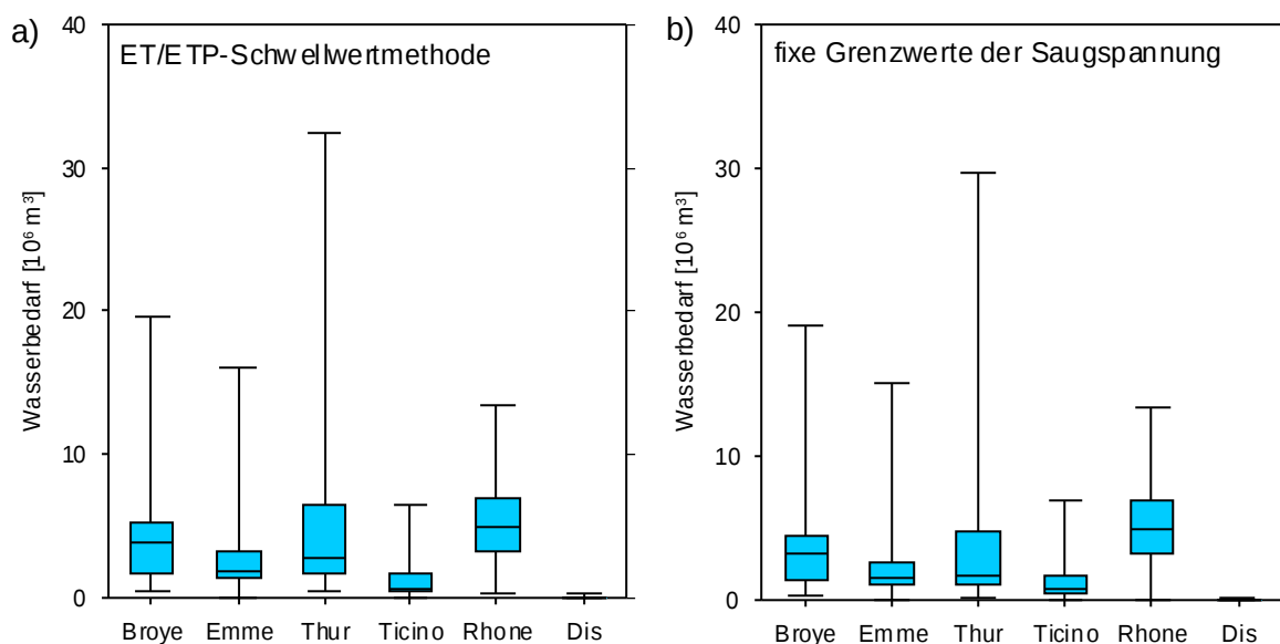
Abbildung 5: Gebietsbezogener saisonaler Bewässerungsbedarf (Spannweite, Median, 1.+ 3. Quartil) für die gesamthaften landwirtschaftlichen Nutzflächen (1980 - 2006), ermittelt a) nach ET/ETP-Schwellwertmethode und b) nach der Methode der fixen Saugspannungsgrenzwerte.
