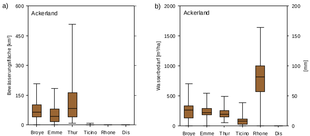
Abbildung 8: Gebietsbezogene saisonale Bewässerungsflächen (links) und zugehöriger Bewässerungsbedarf pro ha (rechts) für Ackerland (jeweils für die Vegetationsperioden des Zeitraumes 1980-2006), ermittelt nach ET/ETP-Schwellwertmethode (Spannweite, Median, 1.+ 3. Quartil).
