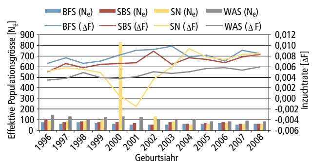
Abb. 4 | Inzuchtrate und effektive Populationsgrösse.
