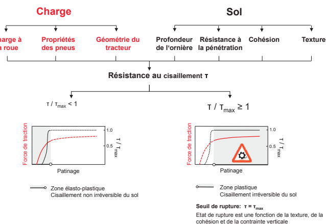
Fig. 4: Deuxième module «Traction, patinage, cisaillement du sol». Principe de base: lorsque les forces de cisaillement générées par les roues sont égales voire supérieures à la résistance du sol au cisaillement, le sol se brise, il y a rupture irréversible.
