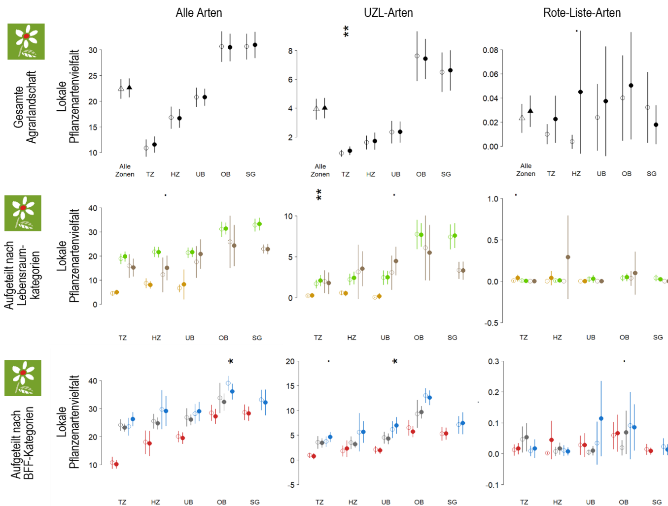
Abbildung 11. Indikator «Lokale Artenvielfalt ( \alpha -Diversität)». Mittlere Anzahl Pflanzenarten pro 10 m 2 . Oben: In der gesamten Agrarlandschaft. Mitte: In der Agrarlandschaft aufgeteilt nach Lebensraumkategorien, gelb – Fruchtfolgeflächen, grün – Grasland, braun – Gehölze. Unten: In der Agrarlandschaft aufgeteilt nach BFF-Kategorien, rot – ausserhalb BFF, grau – BFF Q1 (erfüllt nur Q1, nicht aber Q2), blau – BFF Q2 (erfüllt Q1 und Q2). Die mittlere UZL-Pflanzenartenzahl findet sich in der Mitte und die mittlere Rote-Liste-Artenzahl rechts. Durchschnitt \pm 95 %-Konfidenzintervall. TZ: Talzone, HZ: Hügellzone, UB: Untere Bergzone (Bergzonen I und II), OB: Obere Bergzone (Bergzonen III und IV), SG: Sömmerungsgebiet. ■ P < 0.1 ; * P < 0.05 ; ** P < 0.01 ; *** P < 0.001 . Offene Symbole: Daten aus 2015–2019, geschlossene Symbole: Daten aus 2020–2024.
