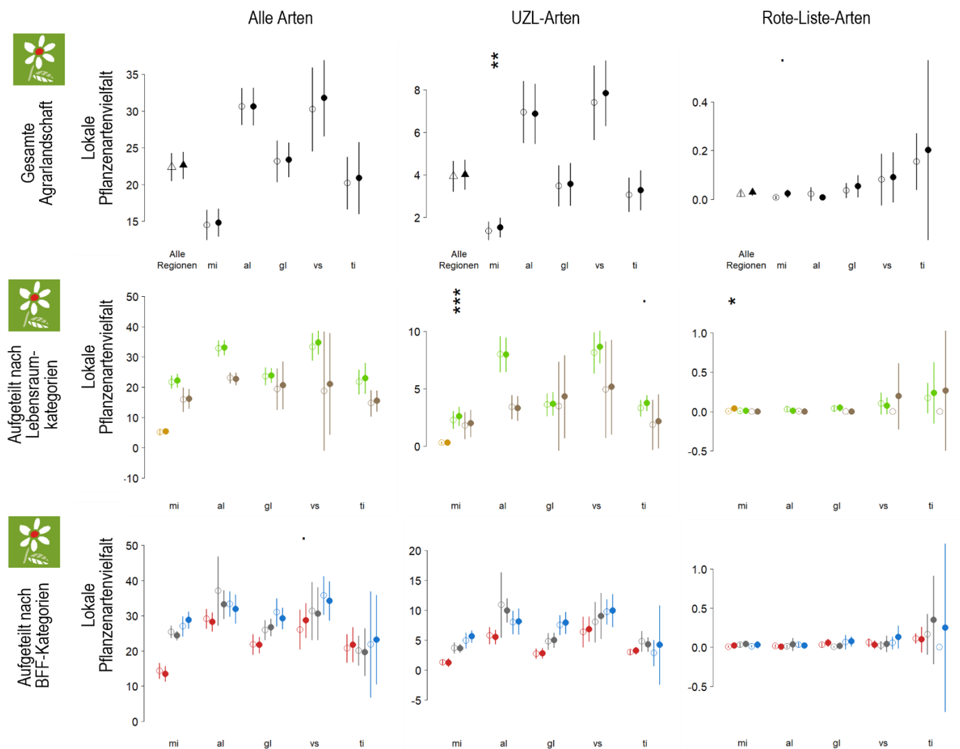
Abbildung A2: Indikator «Lokale Artenvielfalt ( \alpha -Diversität)». Mittlere Anzahl Pflanzenarten pro 10\text{ m}^2 . Oben: In der gesamten Agrarlandschaft pro Untersuchungsquadrat. Mitte: In der Agrarlandschaft aufgeteilt nach Lebensraumkategorien, gelb – Fruchtfolgeflächen, grün – Grasland, braun – Gehölze. Unten: In der Agrarlandschaft aufgeteilt nach BFF-Kategorien, rot – ausserhalb BFF, grau – BFF Q1 (erfüllt nur Q1, nicht aber Q2), blau – BFF Q2 (erfüllt Q1 und Q2). Die mittlere UZL-Pflanzenartenzahl findet sich in der Mitte und die mittlere Rote-Liste-Artenzahl rechts. Durchschnitt \pm 95 %-Konfidenzintervall. mi: Mittelland, tiefe Lagen Jura, Talböden nördlicher Alpenrand, al: Alpen, gl: Hoher, westlicher Jura, tiefe Lagen in den Alpen, vs: Tiefe Lagen Wallis, ti: Südlicher Alpenrand. ■ P < 0.1 ; * P < 0.05 ; ** P < 0.01 ; *** P < 0.001 . Offene Symbole: Daten aus 2015–2019, geschlossene Symbole: Daten aus 2020–2024.
