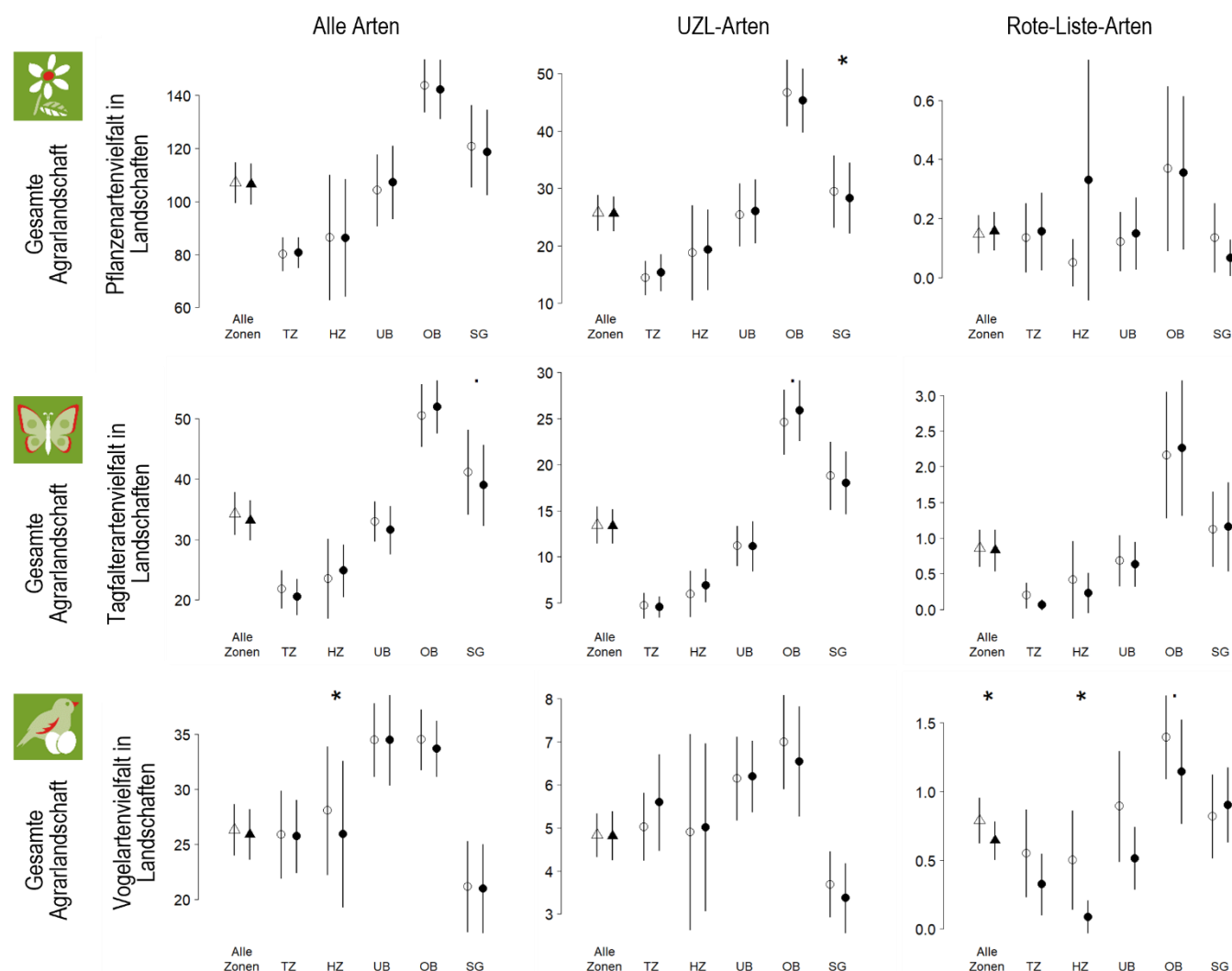
Abbildung 10. Indikator «Artenvielfalt in Landschaften (γ-Diversität)». Oben: Anzahl Pflanzenarten in der gesamten Agrarlandschaft pro Untersuchungsquadrat. Mitte: Anzahl Tagfalterarten in der gesamten Agrarlandschaft pro Untersuchungsquadrat. Unten: Anzahl Brutvogelarten in der gesamten Agrarlandschaft pro Untersuchungsquadrat. Links: Jeweils für alle Arten insgesamt. Mitte: Nur in Bezug auf die UZL-Arten. Rechts: Nur in Bezug auf die Rote-Liste-Arten. Durchschnitt \pm 95 %-Konfidenzintervall. TZ: Talzone, HZ: Hügelizeone, UB: Untere Bergzone (Bergzonen I und II), OB: Obere Bergzone (Bergzonen III und IV), SG: Sömmerungsgebiet. ■ P < 0.1 ; * P < 0.05 ; ** P < 0.01 ; *** P < 0.001 . Offene Symbole: Daten aus 2015–2019, geschlossene Symbole: Daten aus 2020–2024.
