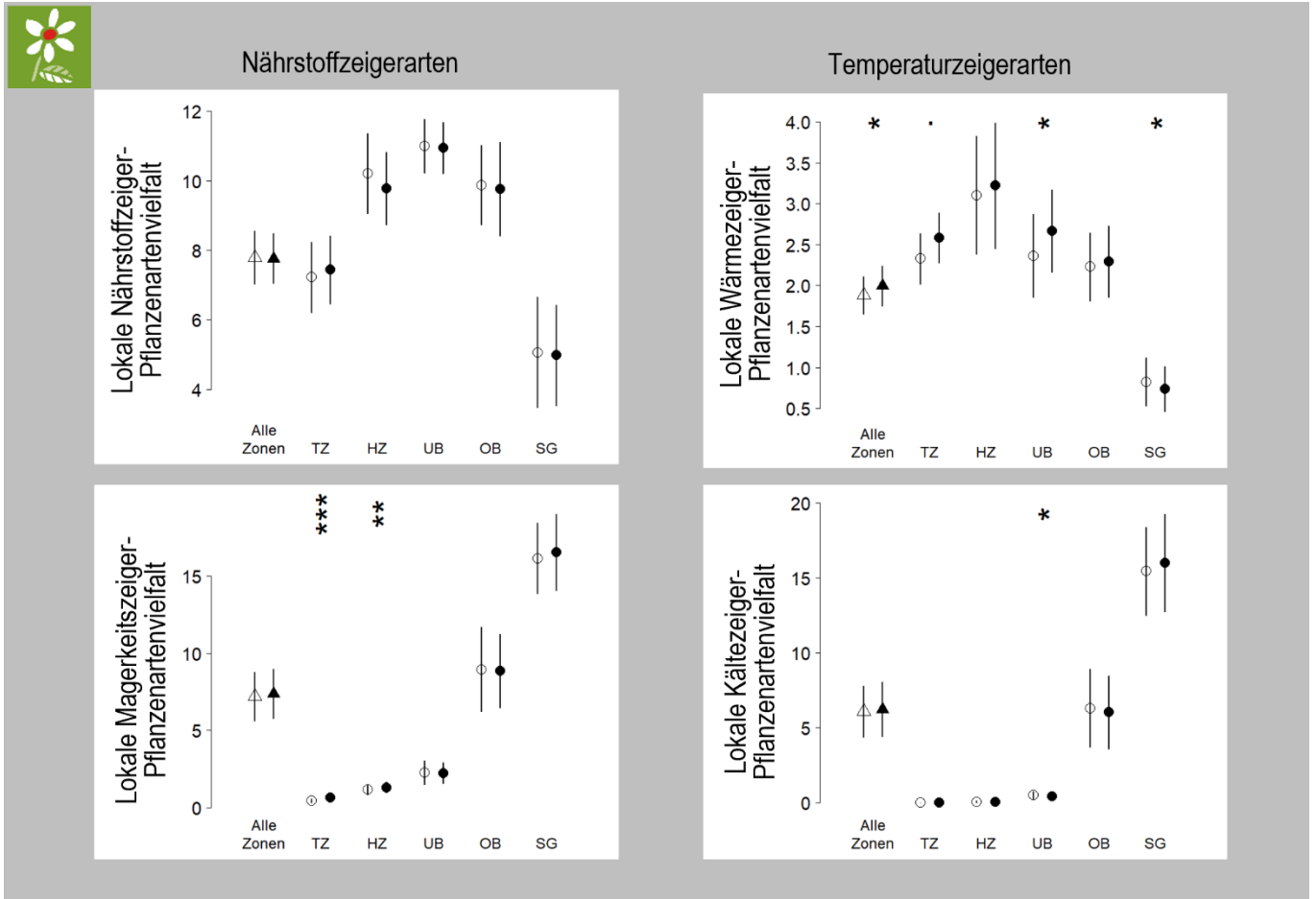
Abbildung 14. Zusatzindikator «Lokale Artenvielfalt ( \alpha -Diversität) von Zeigerarten»: Links oben: Mittlere Anzahl Nährstoffzeigerarten pro 10 m 2 in der gesamten Agrarlandschaft pro Untersuchungsquadrat (Pflanzenarten mit Nährstoffzeigerwert N \geq 4 ). Links unten: Mittlere Anzahl Magerkeitszeigerarten pro 10 m 2 in der gesamten Agrarlandschaft (Pflanzenarten mit Nährstoffzeigerwert N \leq 2 ). Rechts oben: Mittlere Anzahl Wärmezeigerarten pro 10 m 2 in der gesamten Agrarlandschaft pro Untersuchungsquadrat (Pflanzenarten mit Wärmezeigerwert T \geq 4 ). Rechts unten: Mittlere Anzahl Kältezeigerarten pro 10 m 2 in der gesamten Agrarlandschaft (Pflanzenarten mit Wärmezeigerwert T \leq 2 ). Durchschnitt \pm 95 %-Konfidenzintervall. TZ: Talzone, HZ: Hügellzone, UB: Untere Bergzone (Bergzonen I und II), OB: Obere Bergzone (Bergzonen III und IV), SG: Sömmerungsgebiet. ■ P < 0.1 ; * P < 0.05 ; ** P < 0.01 ; *** P < 0.001 . Offene Symbole: Daten aus 2015–2019, geschlossene Symbole: Daten aus 2020–2024.
