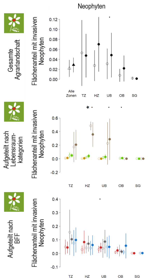
Abbildung 15. Indikator «Invasive Neophyten». Anteil Probeflächen mit invasiven Neophyten. Oben: In der gesamten Agrarlandschaft pro Untersuchungsquadrat. Mitte: In der Agrarlandschaft aufgeteilt nach Lebensraumkategorien, gelb – Fruchtfolgefleichen, grün – Grasland, braun – Gehölze. Unten: In der Agrarlandschaft aufgeteilt nach BFF-Kategorien, gelb – ausserhalb BFF, grau – BFF Q1 (erfüllt nur Q1, nicht aber Q2), blau – BFF Q2 (erfüllt Q1 und Q2). Durchschnitt \pm 95 %-Konfidenzintervall. TZ: Talzone, HZ: Hügelzone, UB: Untere Bergzone (Bergzonen I und II), OB: Obere Bergzone (Bergzonen III und IV), SG: Sömmerungsgebiet. ■ P < 0.1 ; * P < 0.05 ; ** P < 0.01 ; *** P < 0.001 . Offene Symbole: Daten aus 2015–2019, geschlossene Symbole: Daten aus 2020–2024.
