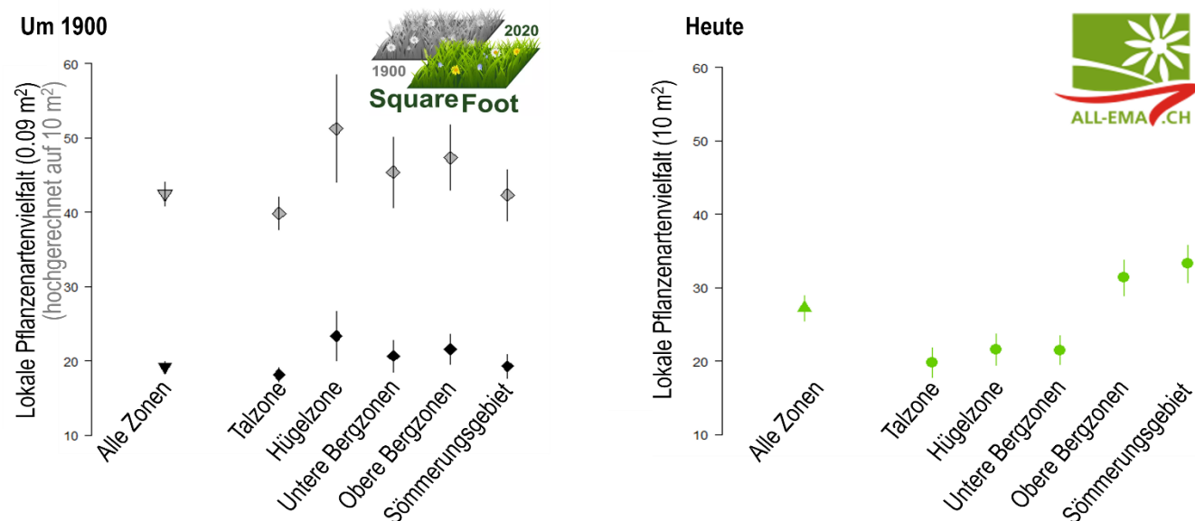
Abbildung 1. Lokale Pflanzenartenvielfalt im Grasland (Durchschnitt \pm 95 %-Konfidenzintervall) in der Schweiz und pro landwirtschaftliche Zone. Links: Erhebungen von 1884–1931, schwarz – Mittlere Anzahl Pflanzenarten pro 1 Quadratfuss = ca. 0.1 m² (Datengrundlage: Riedel et al., 2023); grau – Hochrechnung 1 für die mittlere Anzahl Pflanzenarten pro 10 m². Rechts: Heute, grün – Mittlere Anzahl Pflanzenarten pro 10 m² (Datengrundlage: ALL-EMA; Erhebungen von 2020–2024).
