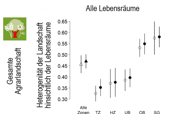
Abbildung 20. Indikator «Heterogenität der Landschaften hinsichtlich der Lebensräume»: Mittlerer Hix-Index basierend auf Lebensräumen in der Agrarlandschaft pro Untersuchungsquadrat. Durchschnitt \pm 95 %-Konfidenzintervall. TZ: Talzone, HZ: Hügelize, UB: Untere Bergzone (Bergzonen I und II), OB: Obere Bergzone (Bergzonen III und IV), SG: Sömmerungsgebiet. ■ P < 0.1 ; * P < 0.05 ; ** P < 0.01 ; *** P < 0.001 . Offene Symbole: Daten aus 2015–2019, geschlossene Symbole: Daten aus 2020–2024.
