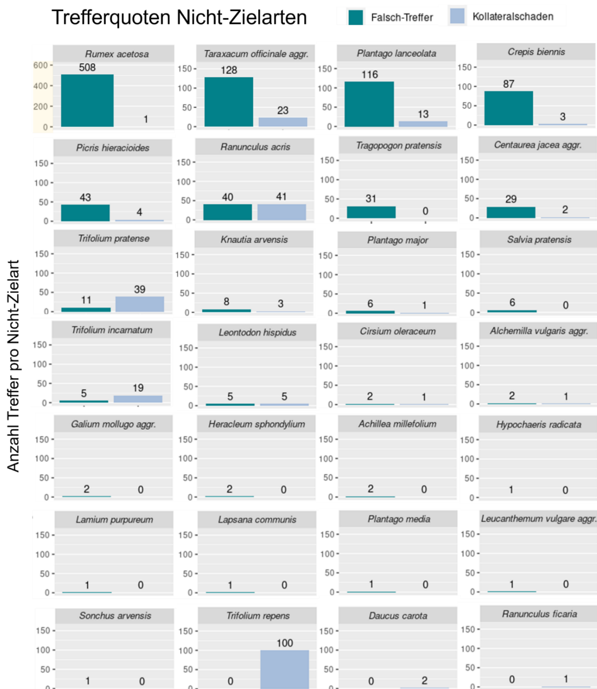
Abbildung 13: Dargestellt werden die absoluten Zahlen pro Art, welche entweder als Falsch-Treffer mit der Wiesenblacke verwechselt wurden, oder als Kollateralschaden im Spritzkegel vom Herbizid getroffen wurden. Die Skala von der Wiesen-Sauerampfer ( Rumex acetosa ) ist angepasst (gelb markiert).
