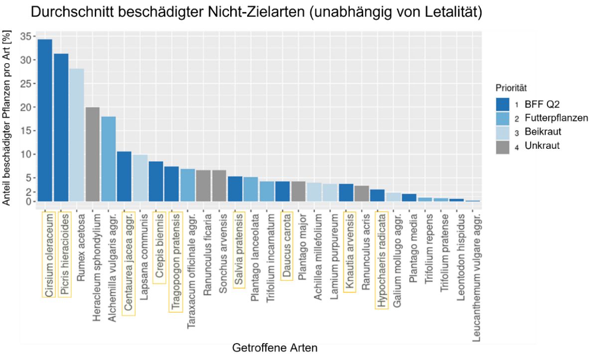
Abbildung 11: Die Barplots zeigen wieviel Prozent einer Nicht-Zielart im Durchschnitt beschädigt wurde (berücksichtigt die mittlere Deckung). Jeder Art wurde eine Priorität 1 (höchste) bis 4 (tiefste) zugeordnet. In Gelb wurden Q2-Zeigerarten markiert, bei welchen mehr als 2% der Individuen beschädigt wurden.
