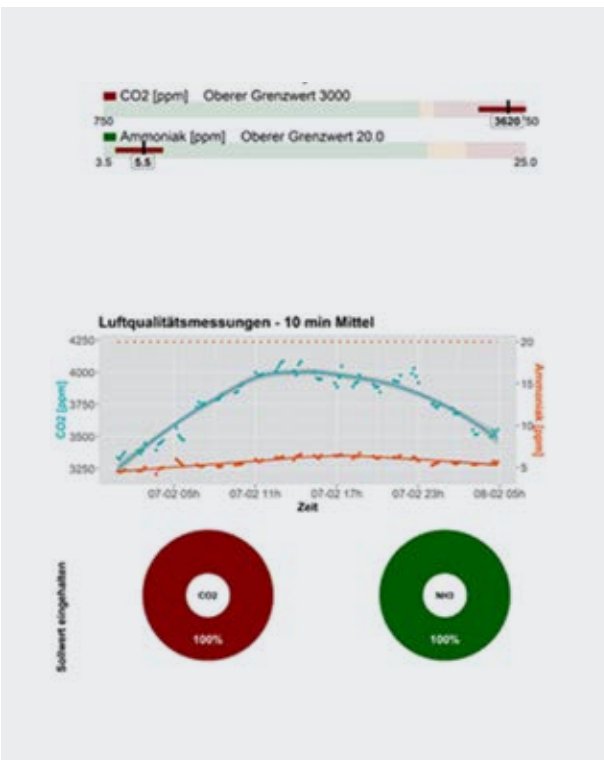
Abbildung 4: Beispiel eines Messberichtes von Kohlendioxid (CO 2 ) und Ammoniak (NH 3 ) über 24 h in einem Broilerstall, Winter, Gasheizung im Stall.
