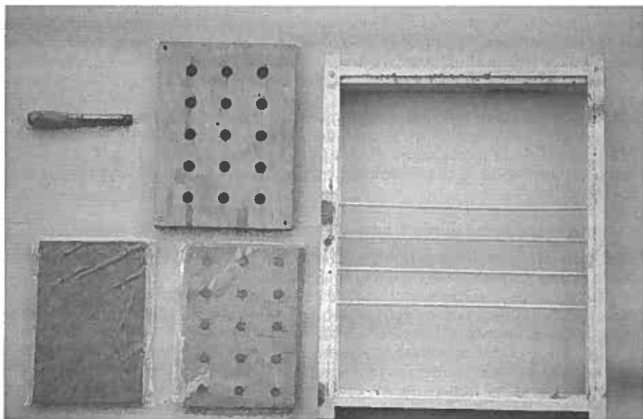
Plaque de Krämer – en bas à gauche, plaque préparée; en bas à droite, plaque perforée; en haut à gauche, emporte-pièce; en haut à droite, chablon de perforation; à droite, cadres en bois pour poser la plaque dans la ruche.
