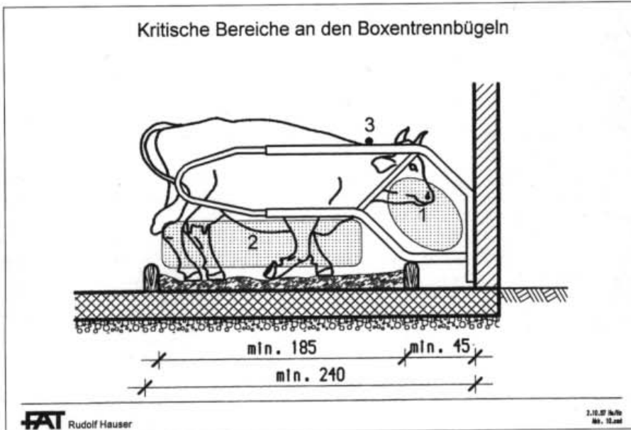
Abb. 10. 1. Beim Aufstehvorgang müssen die Tiere im Kopfbereich seitlich ausweichen können. 2. Die Höhe der seitlichen Abtrennung muss ein Strecken der Beine ermöglichen, aber auch verhindern, dass die Tiere mit dem Rücken darunter rutschen. 3. Das Nackenrohr soll so eingestellt sein, dass die stehende Kuh den Liegebereich nicht verkotet (Masse in cm).
