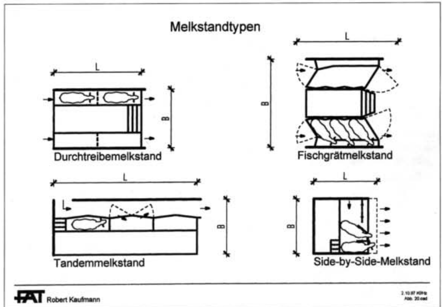
Abb. 20. Übersicht der gebräuchlichsten Melkstandtypen. Im Tandemmelkstand können die Tiere individuell ein- und ausgelassen werden. Tandem- und Durchtreibemelkstand ermöglichen die beste Tierbeobachtung während des Melkens. Der Side-by-Side oder Parallelmelkstand besticht durch den geringen Platzbedarf. Beim Fischgrätmelkstand wird häufig die Melkstanderweiterung provisorisch eingeplant (L = Länge, B = Breite; vgl. Tab. 3).
