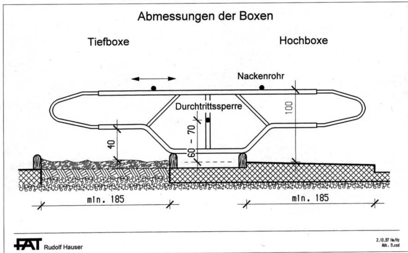
Abb. 9. Bei Tiefboxen bildet eine Strohmatratze eine weiche und verformbare Unterlage. In der Hochboxe ist der Boden mit einer leicht eingestreuten Gummimatte versehen (Masse in cm).
