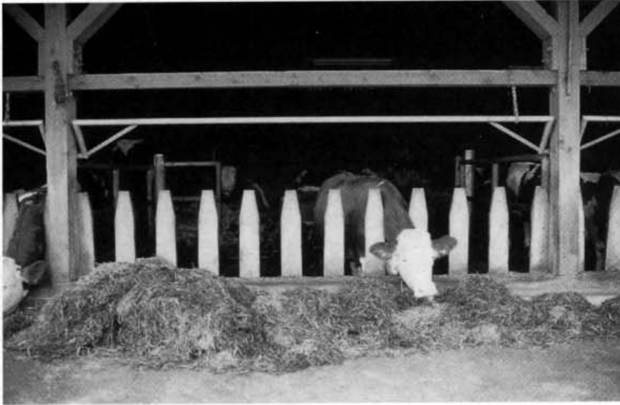
Abb. 16. Mittels eines horizontal liegenden, in der Höhe verstellbaren Rohres können die Kühe auch bei einfachen Palisadenfressgittern gruppenweise eingesperrt werden.
