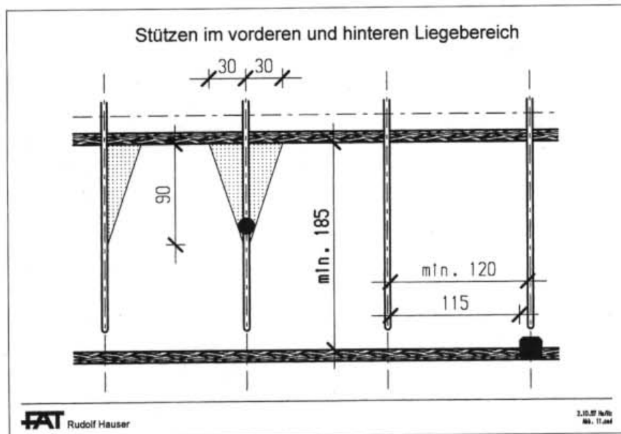
Abb. 11. Einschränkende Stützen in den Boxen sollen nur bei Umbauten toleriert werden. Die angegebenen Masse sind zu beachten (Masse in cm).
