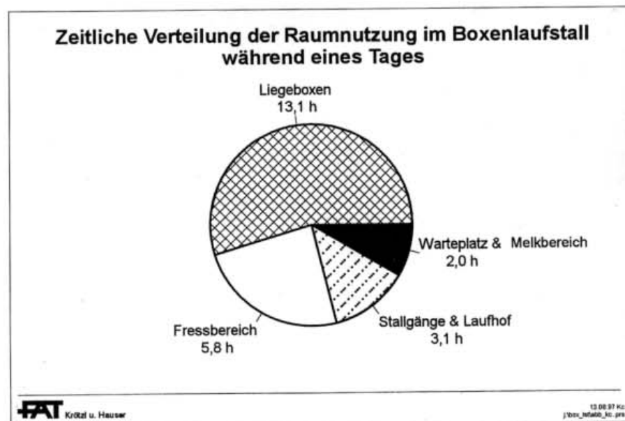
Abb. 3. Die Kuh verbringt mehr als die Hälfte der Zeit im Liegen. Die Gestaltung des Liegebereichs ist daher wichtig (Krötzel und Hauser 1997).
