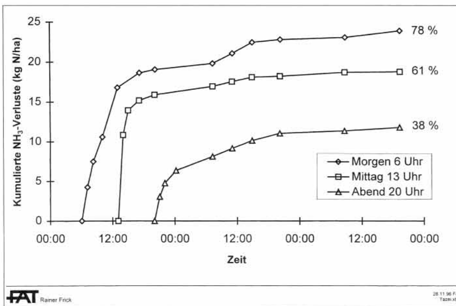
Abb. 2. Kumulierte Ammoniakverluste nach Ausbringung von Rindvieh-Vollgülle ( 33 \text{ m}^3 \text{ pro ha} ) auf Kunstwiese zu drei verschiedenen Tageszeiten. Tänikon, August 1993. Die Prozentwerte entsprechen dem relativen Ammoniakverlust zur ausgebrachten Ammonium-N-Menge. Versuchsbeschreibung siehe Katz 1996.
