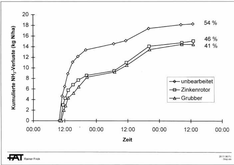
Abb. 6. Kumulierte Ammoniakverluste in den ersten zwei Tagen nach Ausbringung von Rindvieh-Vollgülle ( 34 \text{ m}^3 \text{ pro ha} ) auf Getreidestoppeln mit unterschiedlicher Bearbeitung vor dem Austrag. T \ddot{a} nikon, August 1992. Die Prozentwerte entsprechen dem relativen Ammoniakverlust zur ausgebrachten Ammonium-N-Menge. Versuchsbeschreibung siehe Katz 1996.
