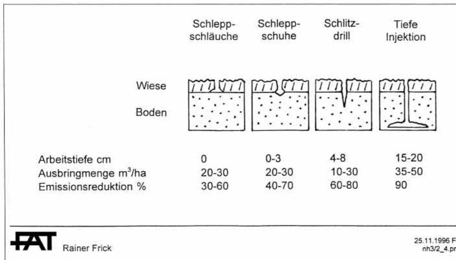
Abb. 7. Arten der Ablage bzw. Einleitung der Gülle bei den verschiedenen Techniken für die verlustarme Gülleausbringung.
