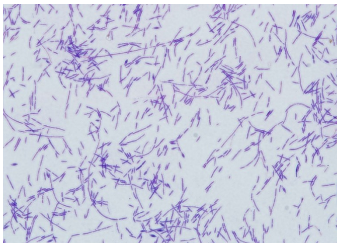
Fig. 1: Vue microscopique de Paenibacillus larvae après coloration Gram. Formation de chaînes. Agrandissement 1000X, (photo : B. Dainat, CRA, Agroscope)
