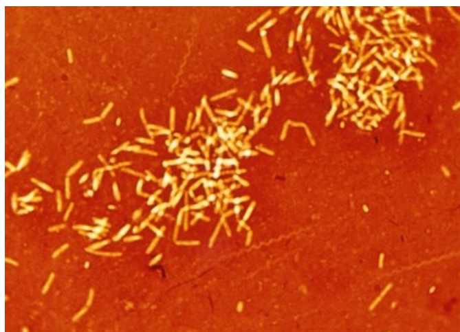
Fig. 2 : Diagnostic au microscope de la loque américaine. Les tresses de flagelles caractéristiques sont visibles. Agrandissement 1000X. (photo : Agroscope).
