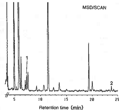
Abb. 1. GC-MS-Chromatogramm der flüchtigen Komponenten (Purge & Trap®-Analysemethoden, im Scan-Modus; Modell HP 5970) in einer aus dem Handel erhältlichen UHT-indirekt-erhitzten Milchprobe.
