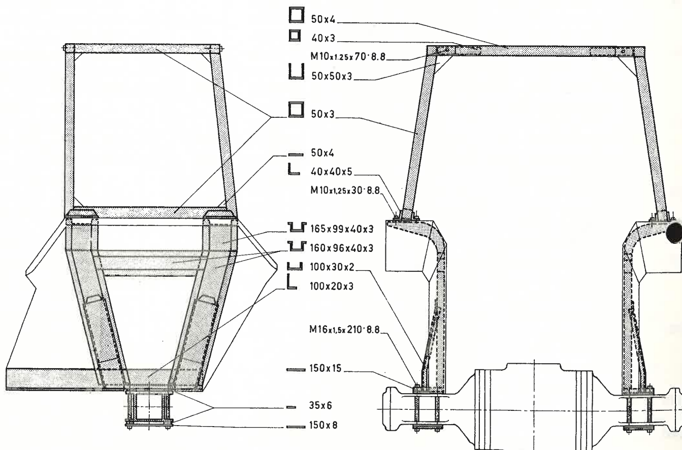
Beispiel eines ausgeführten Sicherheitsrahmens für Traktoren
