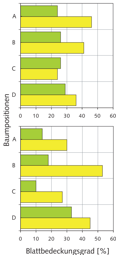
Abb. 5: Oben: Mit zwei FAT-Lamellenprüfständen kann die Grundeinstellung des Sprühgerätes auf die Baumform optimiert werden. Links: Beispiele der vertikalen Wasserverteilung. Rechts: Obwohl im Oberbereich weniger Wassermenge eingestellt war, weisen praktisch alle Baumpositionen einen guten oder einen heterogenen (mit/ohne Gebläseaufsatz) Blattbedeckungsgrad auf.
