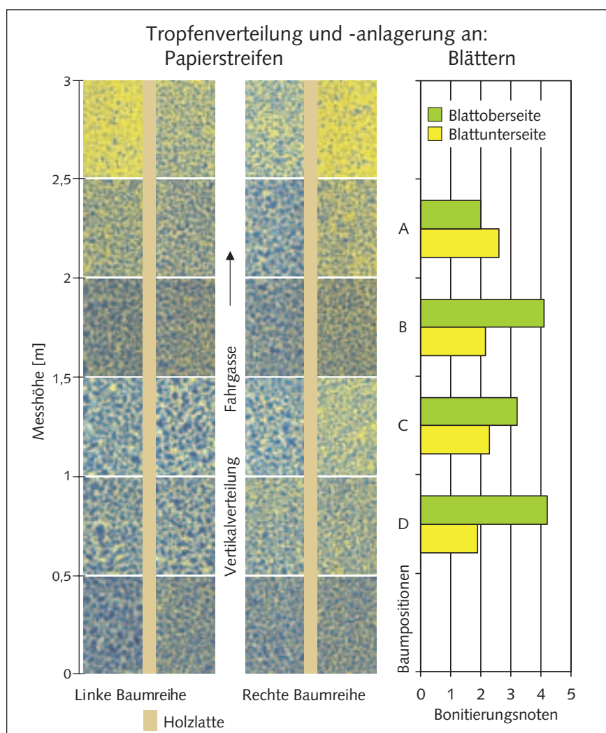
Abb. 8: Vertikalverteilung und Tropfenanlagerung an Blättern (Fischer).
