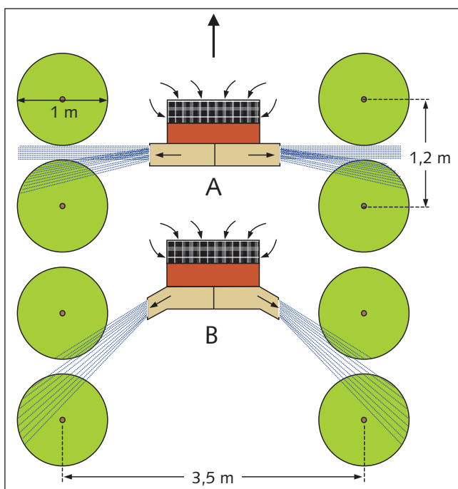
Abb. 10: Schema der Arbeitsweise des Sprühgerätes mit Umkehraxialgebläse: A = Bei 90° Ausblaswinkel zur Fahrtrichtung gelangt ein Teil der Brühe unkontrolliert durch die Leerstellen in die benachbarten Fahrgassen. B = Bei 40 bis 45° schrägen Ausblaswinkeln nach hinten hingegen werden die Tropfen durch das Blattwerk aufgenommen.
