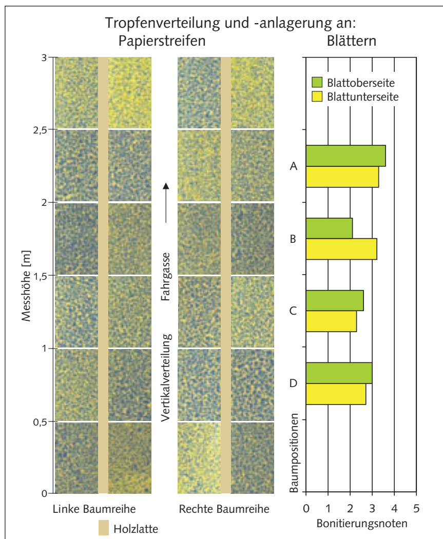
Abb. 7: a) Vertikalverteilung und Tropfenanlagerung an Blättern (Tifone).
