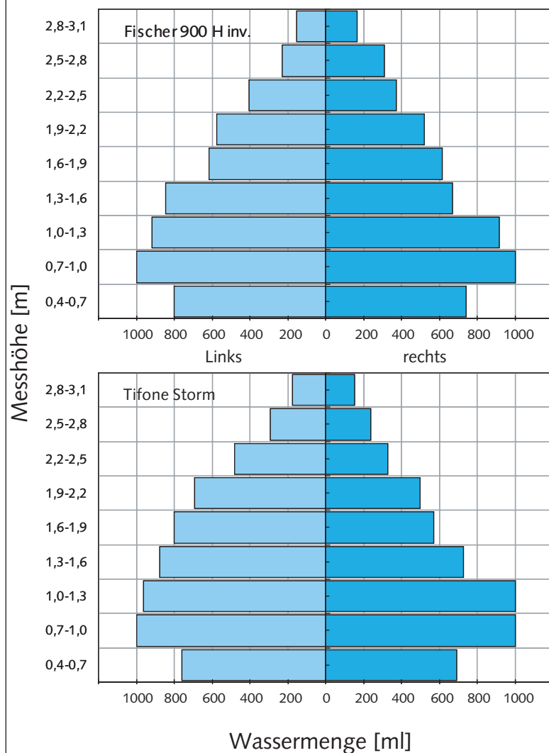
Abb. 5: Oben: Mit zwei FAT-Lamellenprüfständen kann die Grundeinstellung des Sprühgerätes auf die Baumform optimiert werden. Links: Beispiele der vertikalen Wasserverteilung. Rechts: Obwohl im Oberbereich weniger Wassermenge eingestellt war, weisen praktisch alle Baumpositionen einen guten oder einen heterogenen (mit/ohne Gebläseaufsatz) Blattbedeckungsgrad auf.
