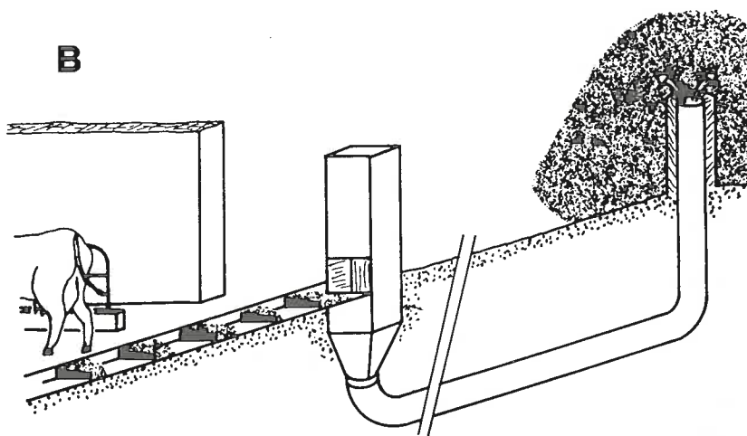
Abb. 4: Maulwurfentmistung: A Horizontal arbeitend mit ebenerdigem Mistplatzausgang; B Vertikal arbeitend mit erhöhtem Mistplatzausgang.
