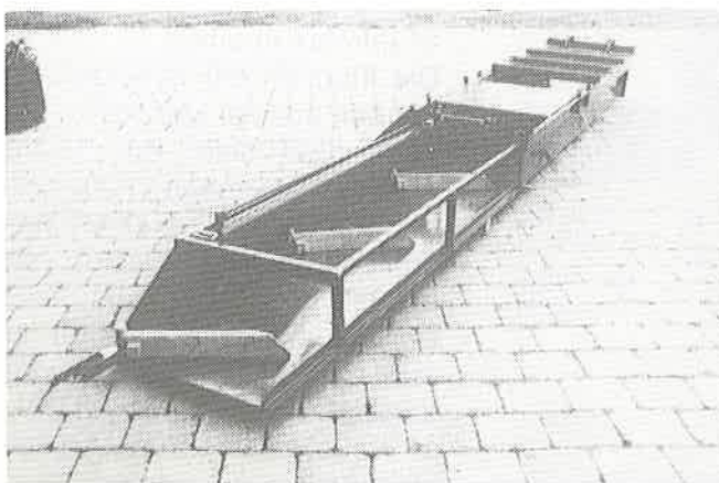
Abb. 2: Die Schubstange endet mit einem verstärkten Schiebeschild in der Druckkammer.
