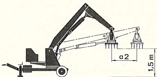
Abb. 20: Breite des Arbeitsfeldes in 1,5 m Höhe
