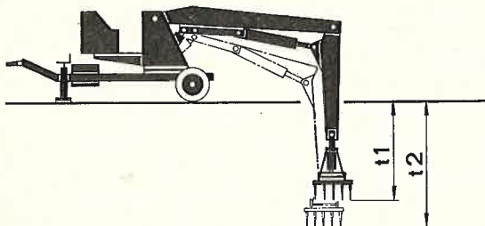
Abb. 17: max. Greiftiefe
