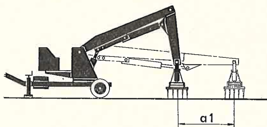
Abb. 19: Breite des Arbeitsfeldes auf Standebene
