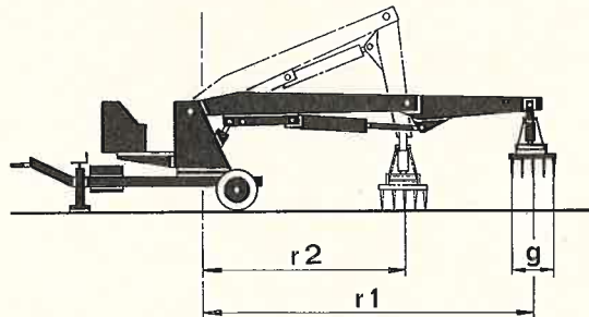
Abb. 18: Reichweite
