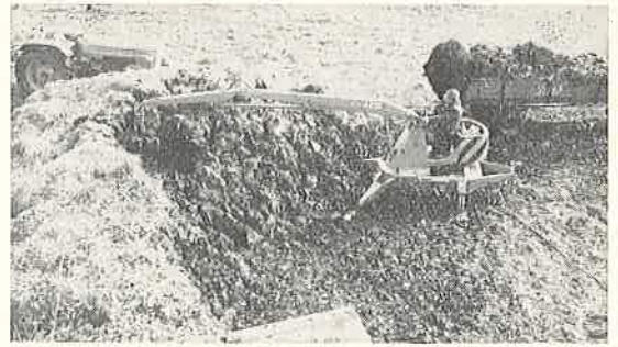
Abb. 12: KMF 417 bei den praktischen Messungen.
