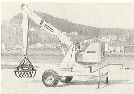
Abb. 5: Kran mit zwei Stützen.
