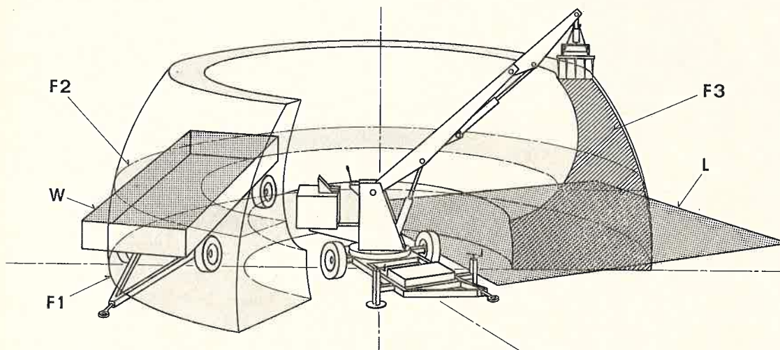
Abb. 1: Arbeitsbereich eines Mistladekrans
