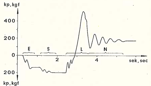
Abb. 13: Verlauf der Kräfte am Mistgreifer;
