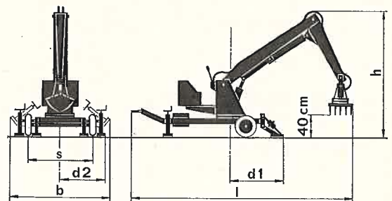
Abb. 14: Hauptabmessungen;
