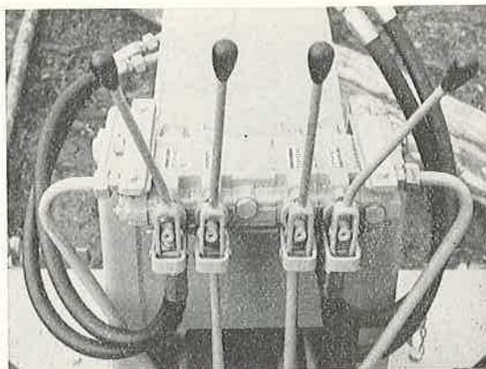
Abb. 10: Uebersichtliche Hebelanordnung mit gut lesbarer Beschriftung.
