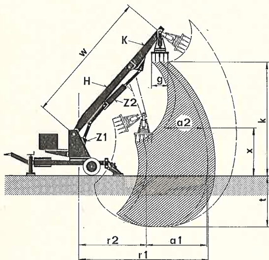
Abb. 2: Vertikales Arbeitsfeld
